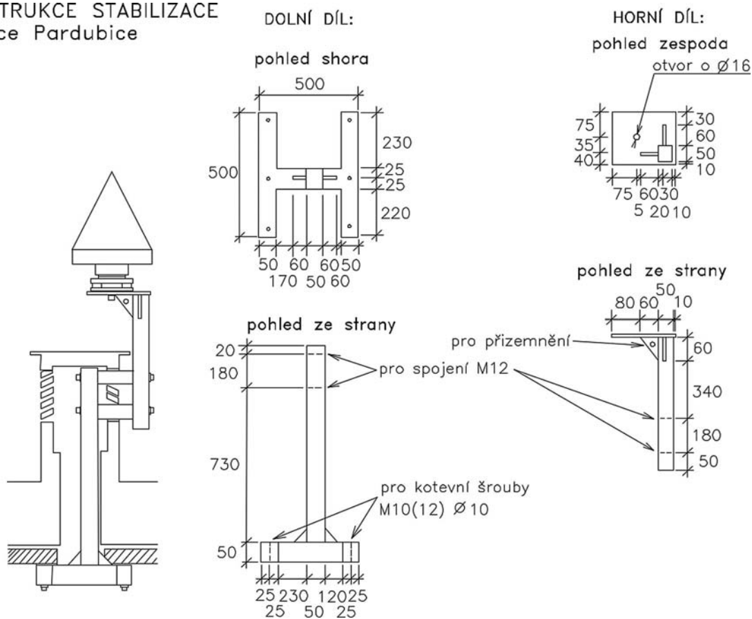
Obr. 2 Zákres konstrukce antény z projektu lokalizace stanice Pardubice
